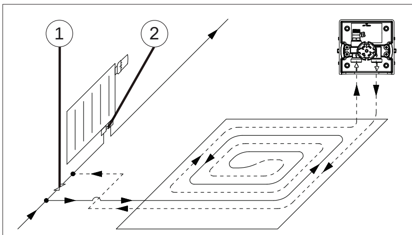
Рис. 19: Подключение с перепускным клапаном и узлом нижнего подключения радиатора с байпасом
